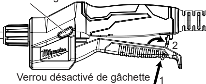
Verrou désactivé de gâchette
